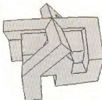
Figure 8 : coordonnées observateur
